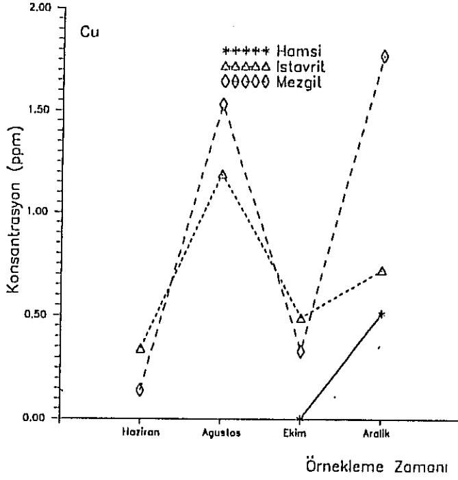
Şekil 4. Değişik örneklenme zamanlarında balıklarda ölçülen bakır konsantrasyonları
